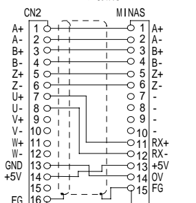
松下電器製MINASシリーズエンコ-ダ接続
